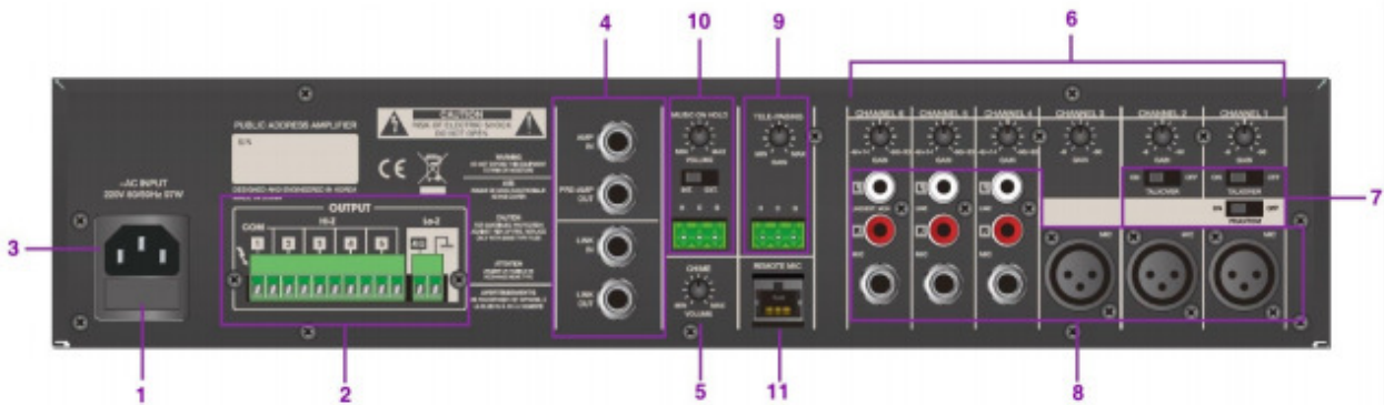
Ilustración 2: Vista Trasera de QX-240
